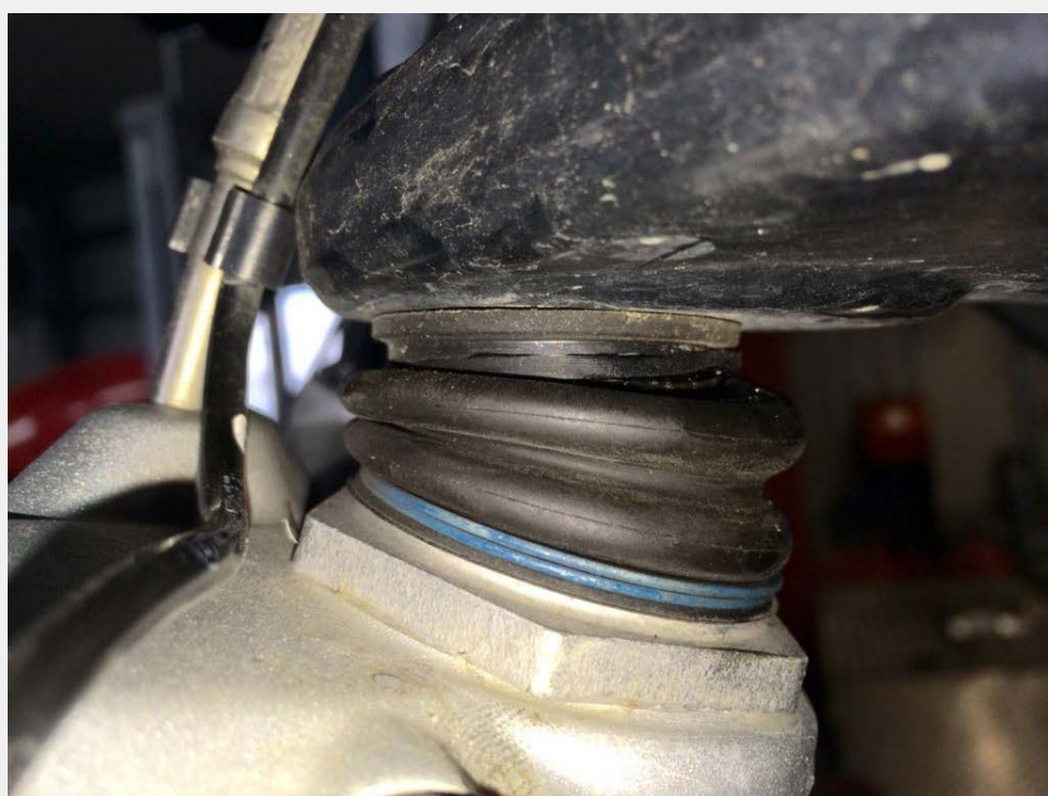
Frisch repariert mit neuem Schutzgummi am Kugelgelenk der BMW R 4 Ventil Telelever Gabel
